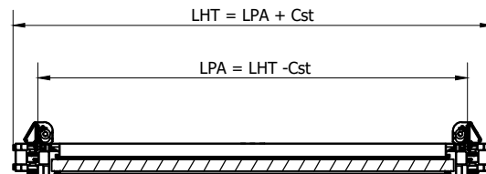
A-A ( 1:10 )
